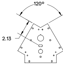
120° Y Bracket
