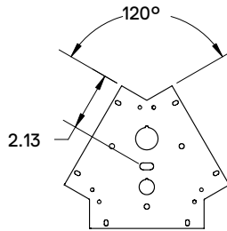
120° Y Bracket
